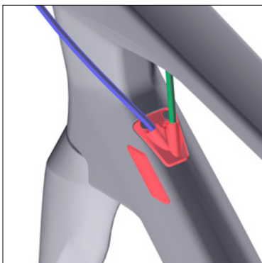
Sortie du logement de la transmission
