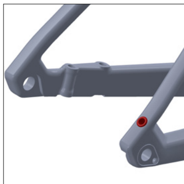
Sortie du câble de dérailleur arrière
